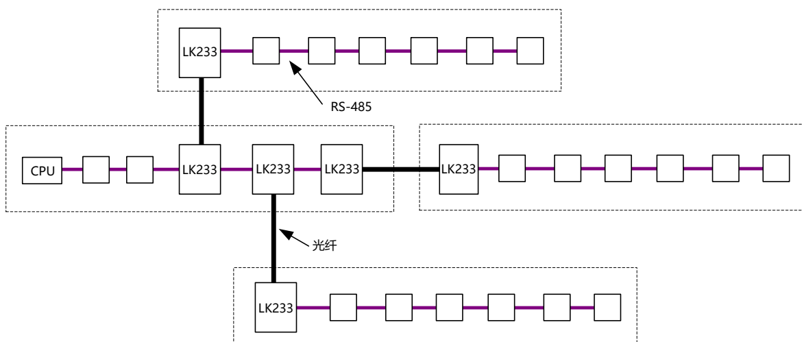
图 215 星型网络结构
