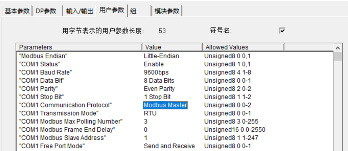
图 228 Modbus 主站参数设置
