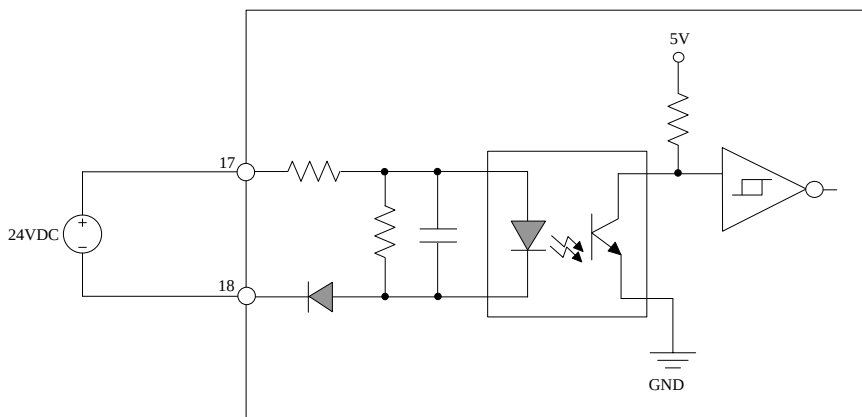
图 86 LK710 现场电源掉电检测电路简图
