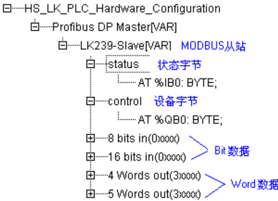
图 258 MODBUS 从站数据列表
