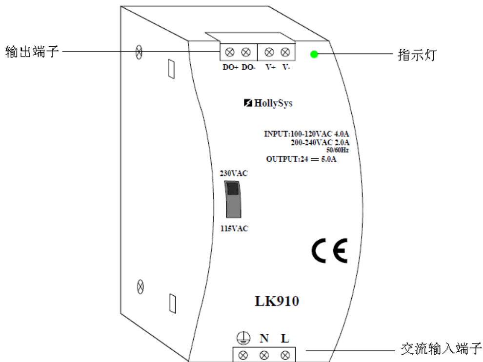
图 310 LK910 模块接线端子和指示灯
