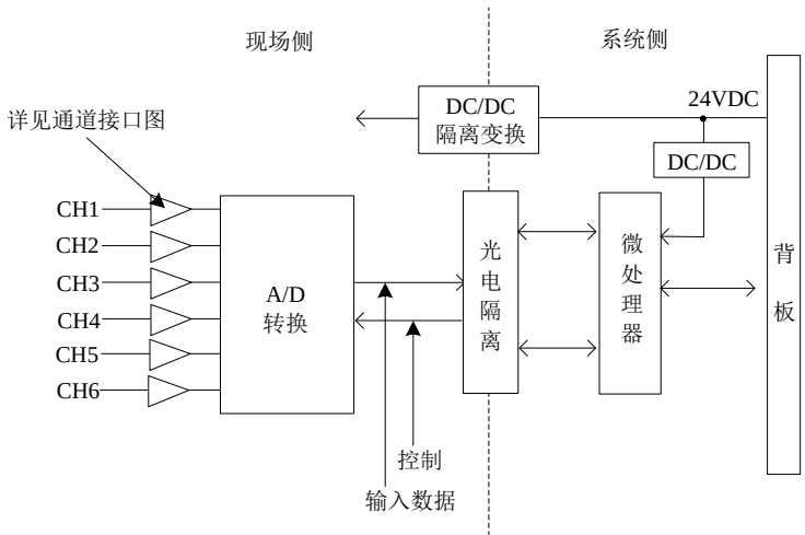
图 121 LK430 内部结构框图
