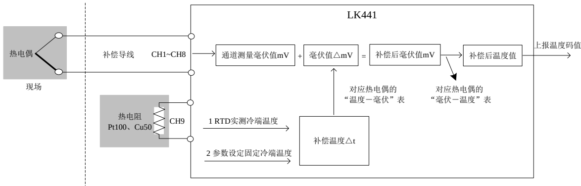
图 134 LK441 冷端温度补偿框图
