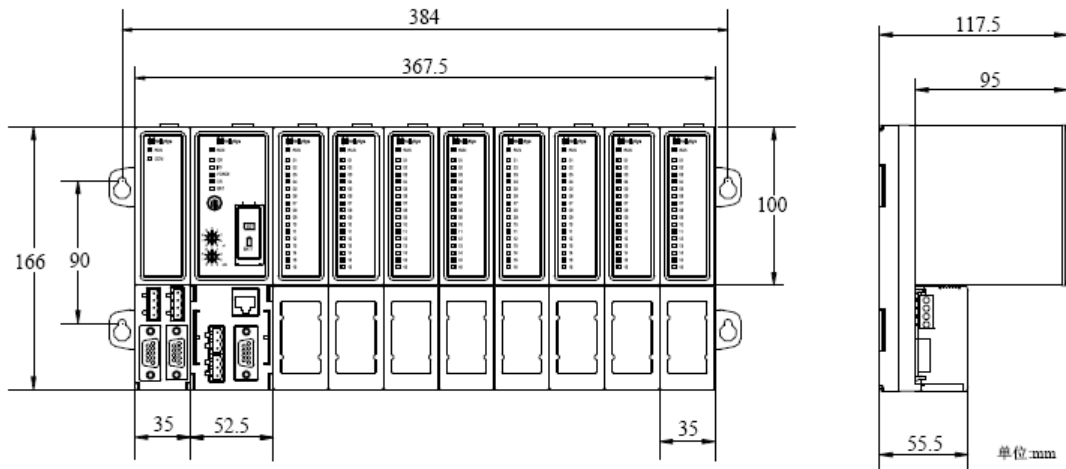
图 293 LK104 背板的安装尺寸
