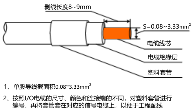
图 34 I/O 电缆的加工要求
