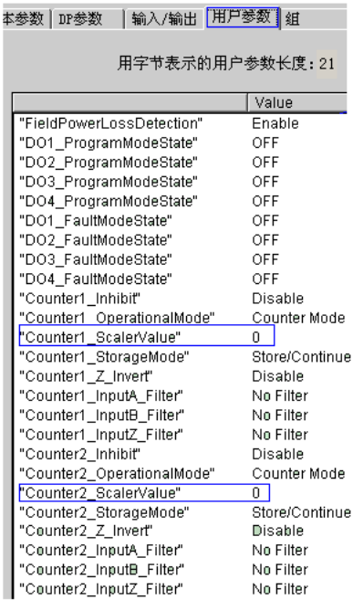
图 170 计数器测频时间设置
