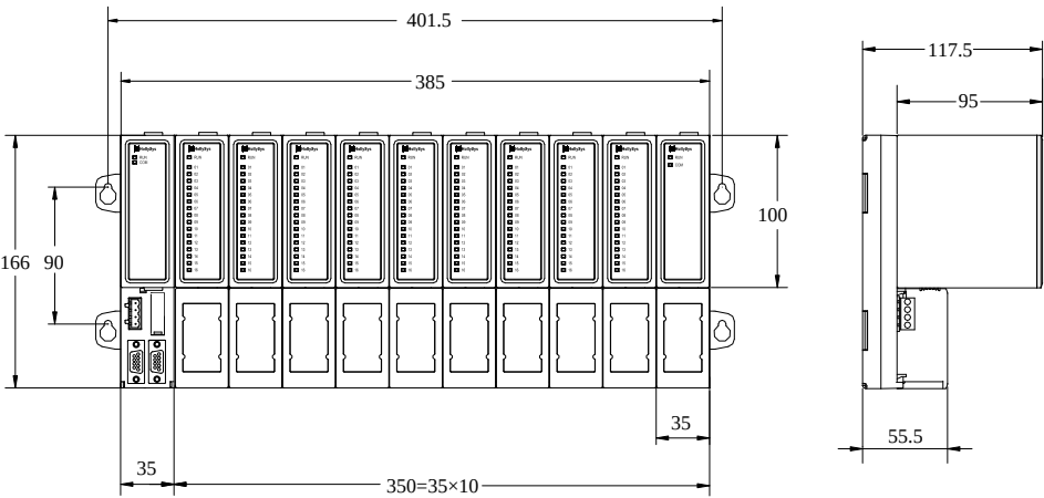
图 309 LK117 背板的安装尺寸
