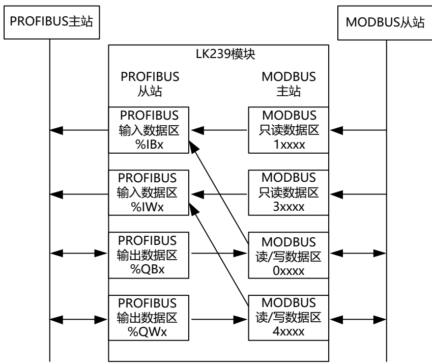
图 244 LK239 作主站时模块的数据交换功能实现简图
