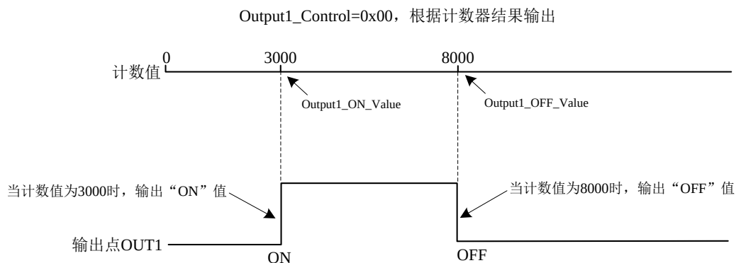
图 171 根据计数结果输出时 OUT1 的输出时序
