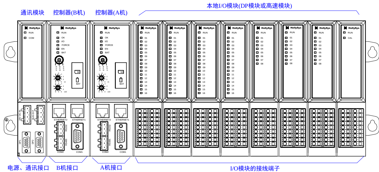
图 299 LK123 背板的前视图
