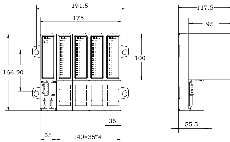
图 308 LK118 背板的安装尺寸
