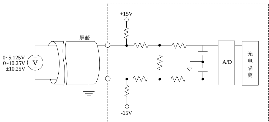
图 95 LK410 通道接口电路图
