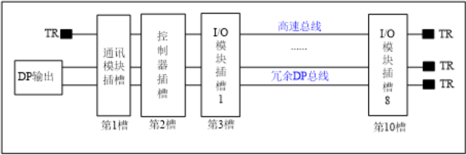
图 296 LK106 本地背板内部结构
