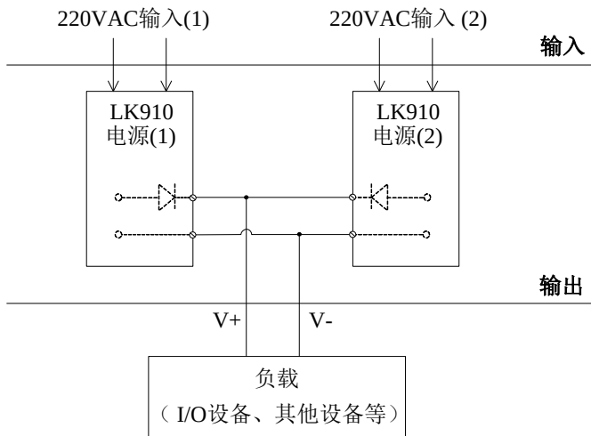
图 313 LK910 电源的冗余配置
