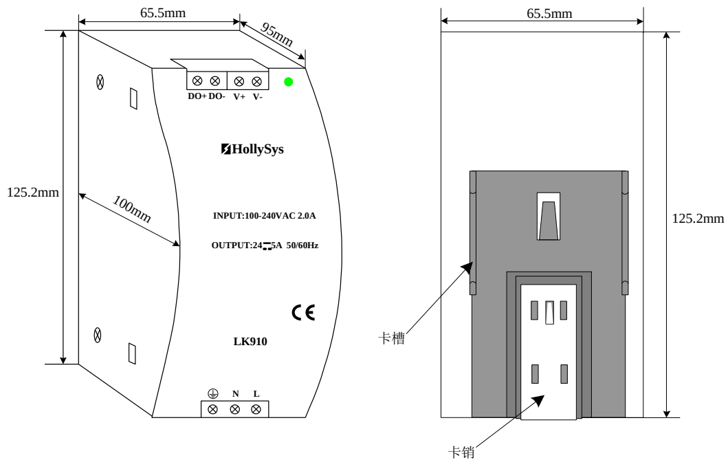
图 315 LK910 电源外观尺寸
