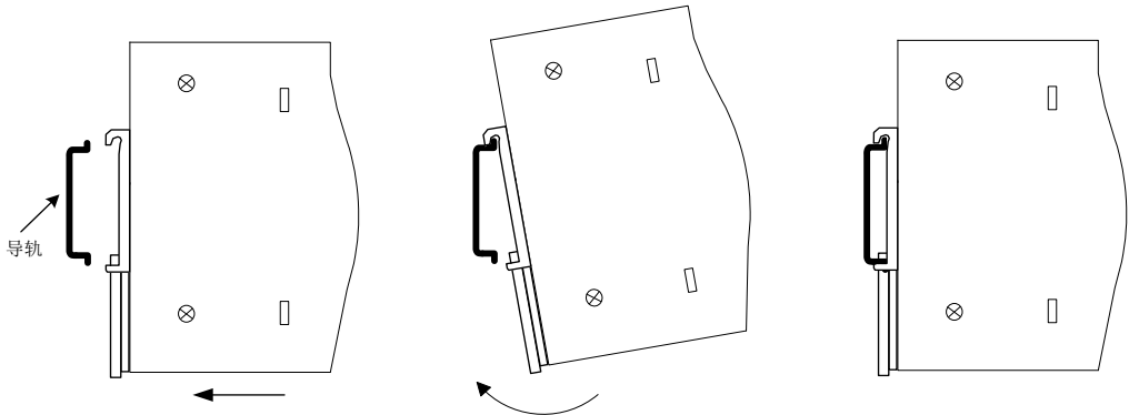
图 314 LK910 电源的安装
