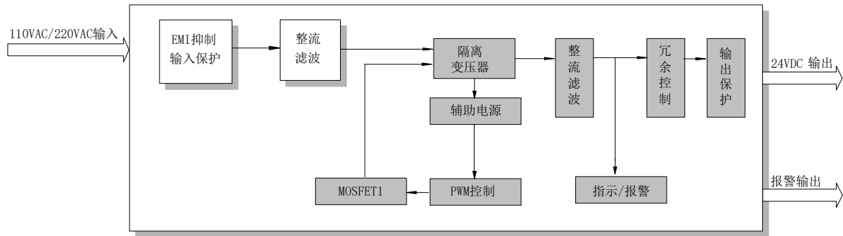
图 311 LK910 电源原理框图
