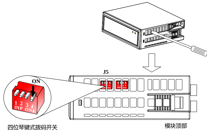
图 212 LK233 拨码开关的设置
