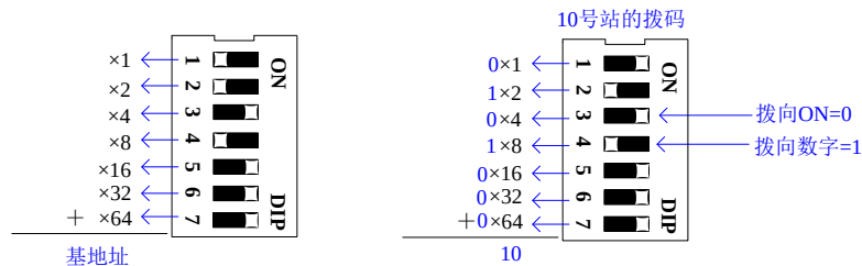
图 307 背板基地址的设定
