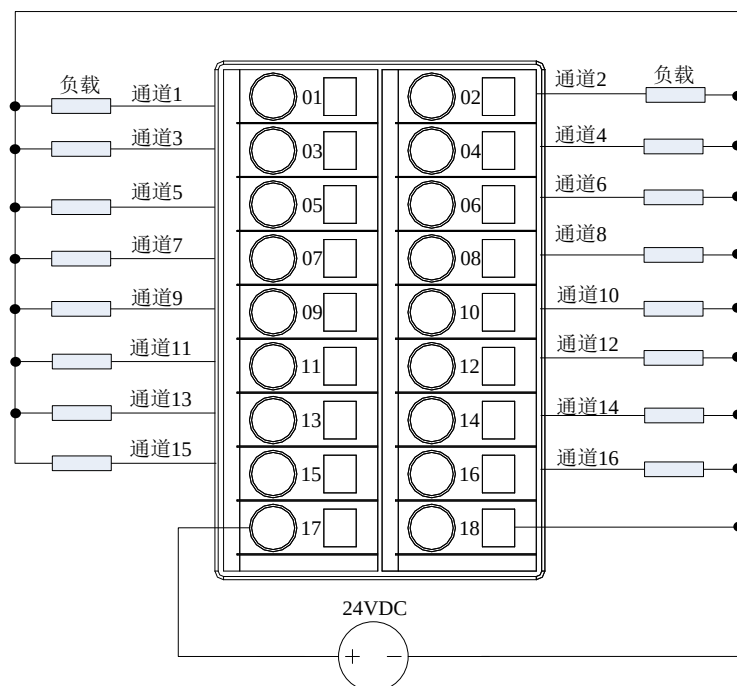
图 84 LK710 对应背板端子接线图
