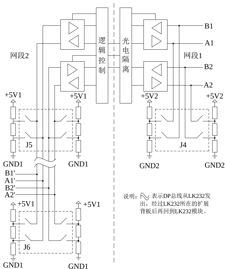
图 203 LK232 安装在扩展背板时的总线转换图
