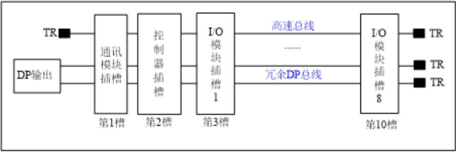
图 292 LK104 本地背板内部结构
