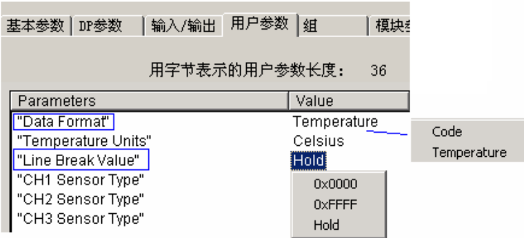
图 126 LK430 断线检测参数设置
