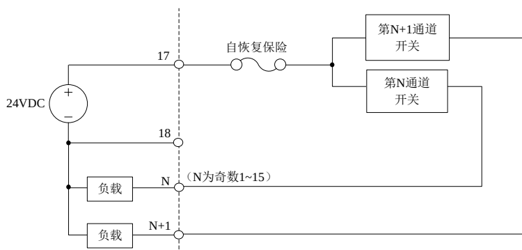
图 85 LK710 通道过流保护电路简图
