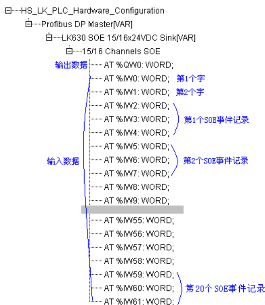
图 199 LK630 的数据区界面
