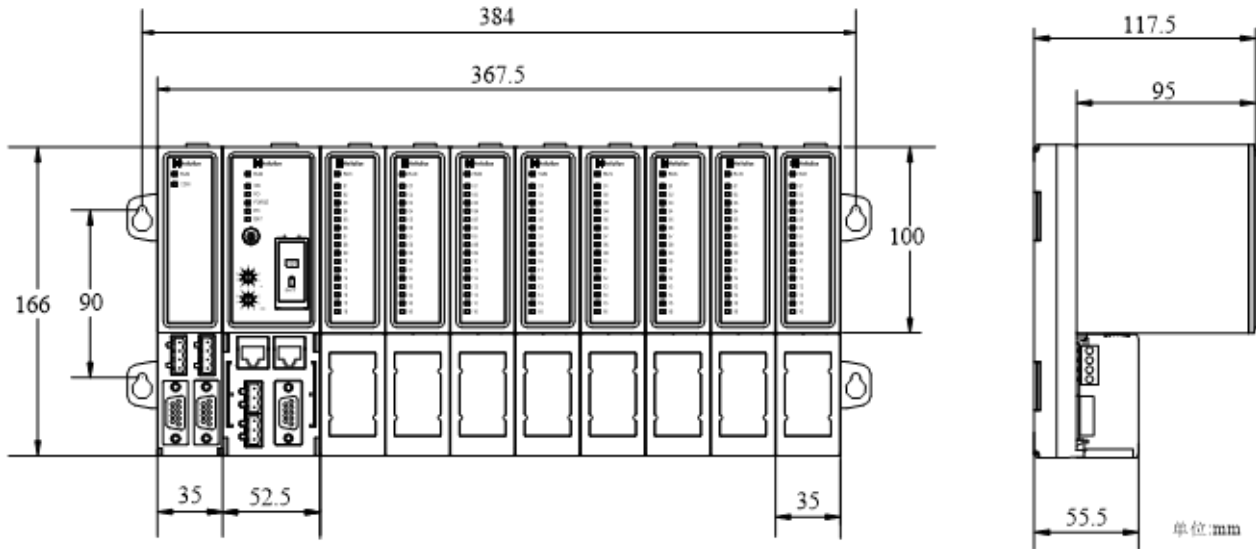
图 297 LK106 背板的安装尺寸
