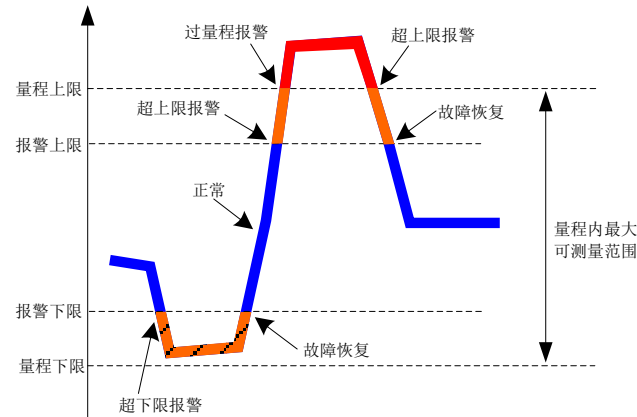
图 136 LK441 超限报警示意图
