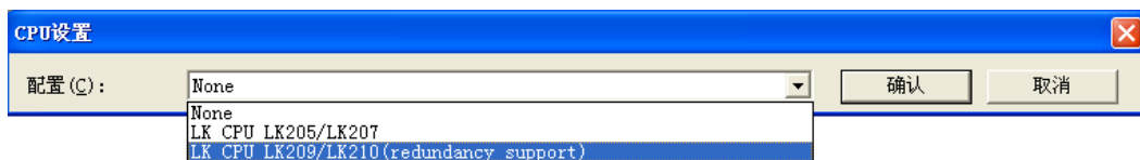
图 37 CPU 设置
