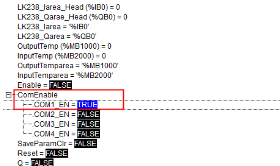
图 238 使能端口
