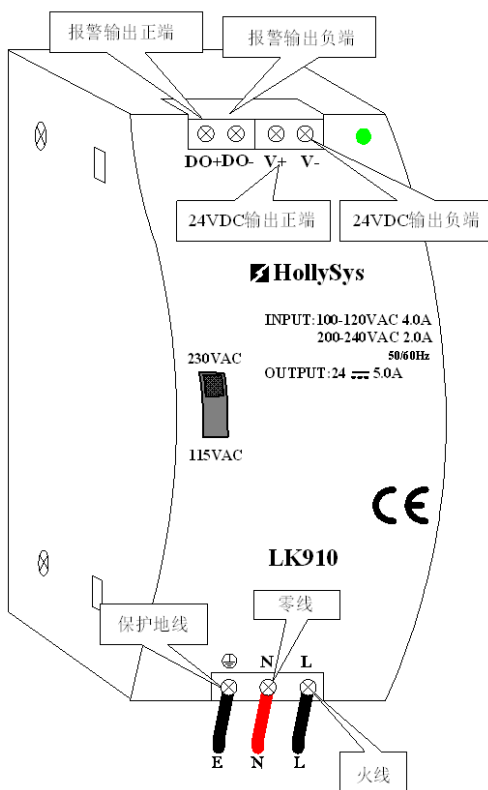
图 312 LK910 电源接线端子说明
