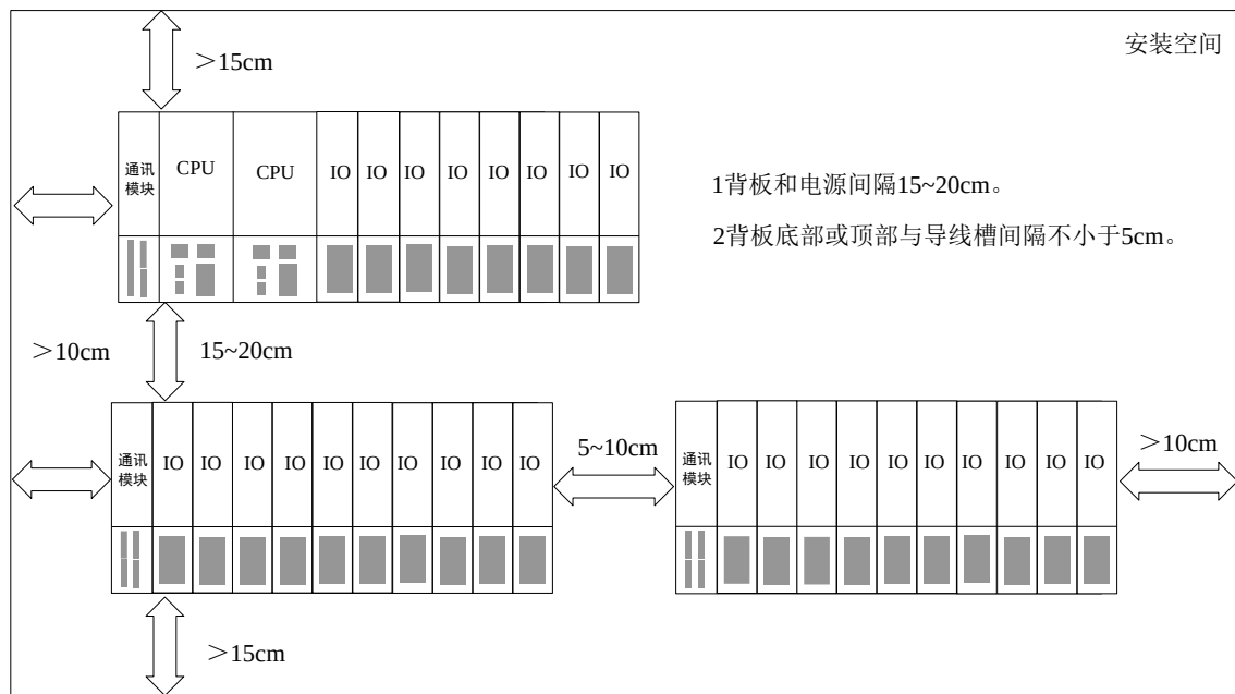
图 14 LK 背板安装的空间布局要求
