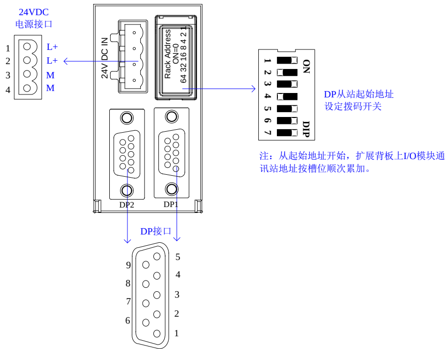
图 305 LK117、LK118 背板的电源和通讯接口
