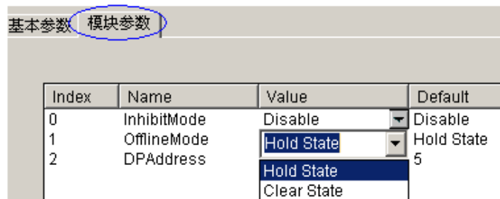
图 288 LK255 的模块参数
