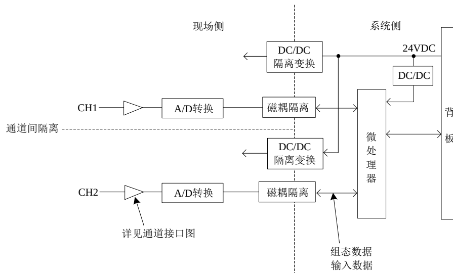
图 110 LK412 模块内部结构框图
