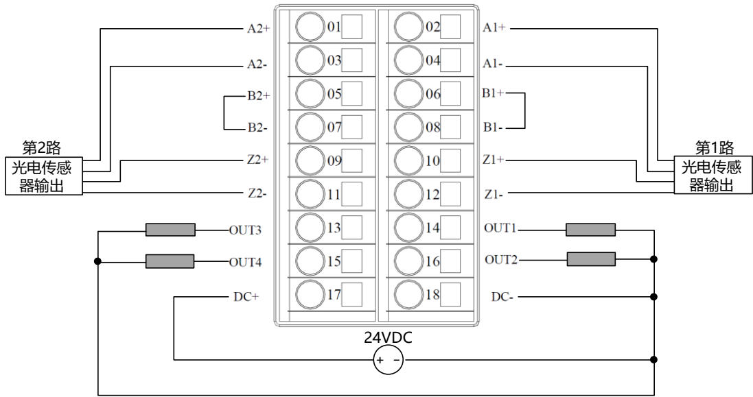
图 167 计数模块与光电传感器的连接
