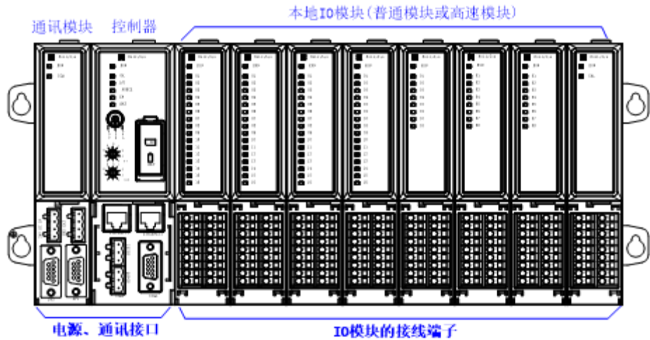
图 295 LK106 本地背板的正视图
