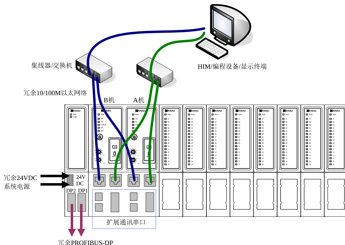
图 68 冗余控制器以太网的连接
