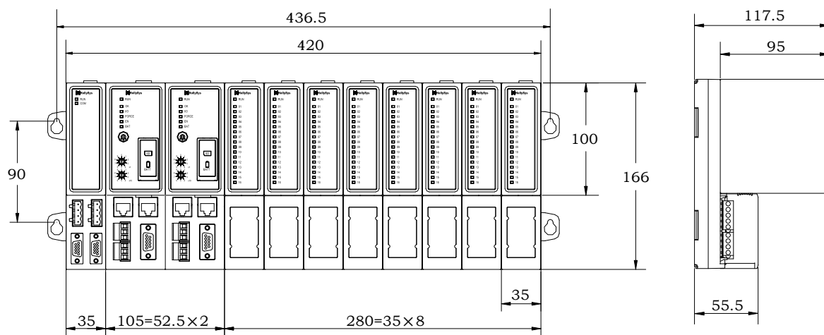
图 301 LK123 背板的安装尺寸
