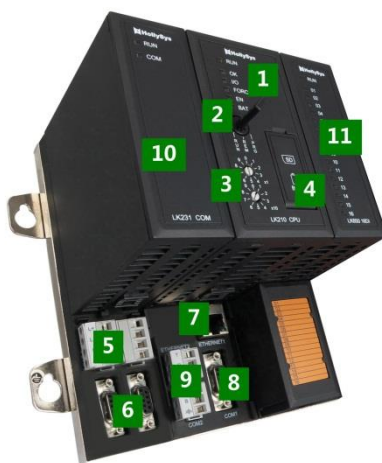
图 1 LK 控制器
