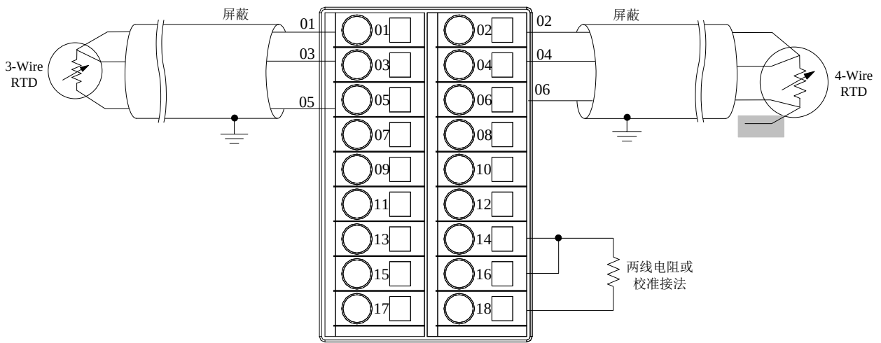
图 123 LK430 背板端子接线示意图
