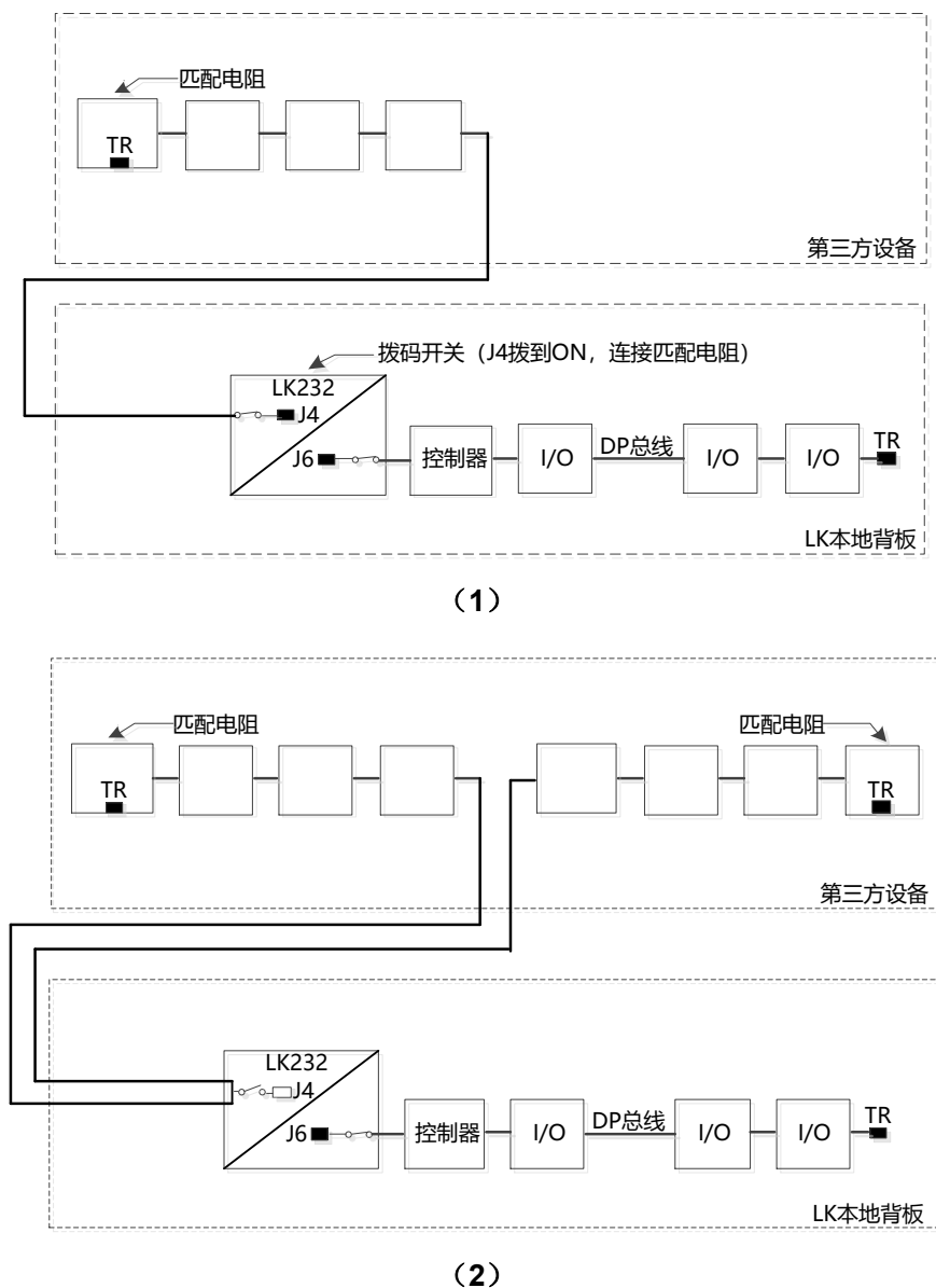
图 33 连接第三方设备时本地背板终端匹配电阻设置
