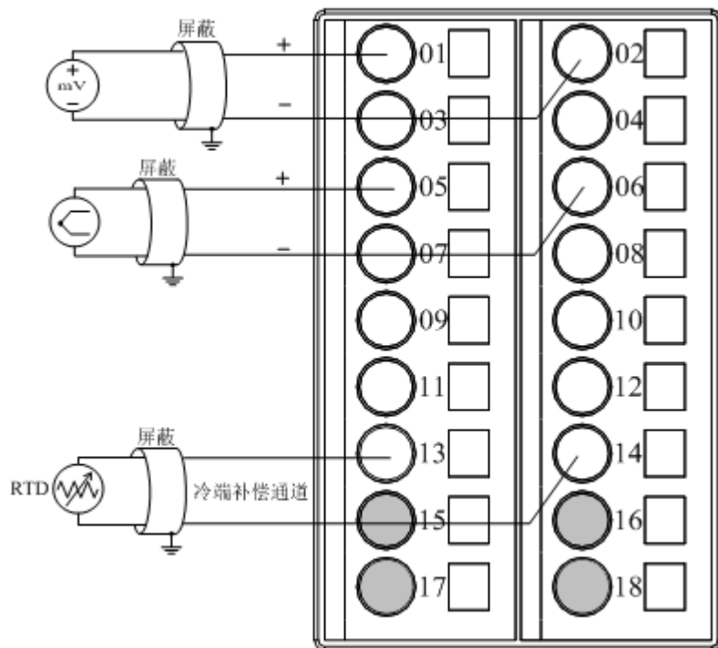
图 140 LK442 背板端子接线图
