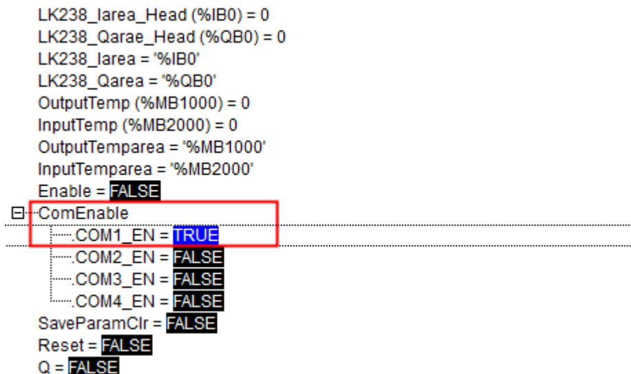
图 234 使能端口
