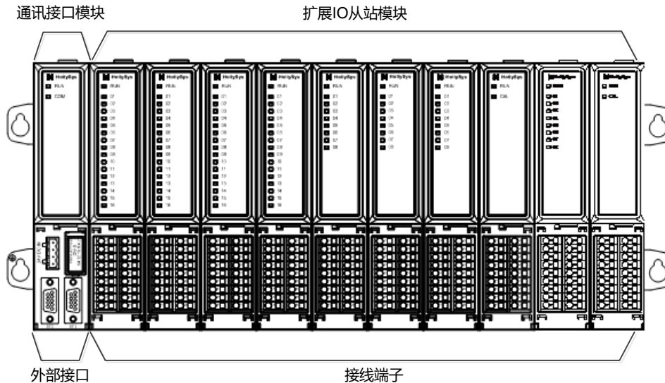
图 303 LK117 背板的结构
