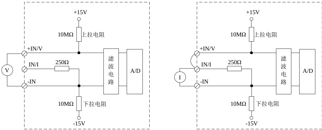
图 120 LK412 通道断线检测电路图
